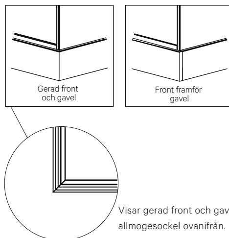
Skarv vid integrerad diskmaskin art.nr. 3889 och 3890.
