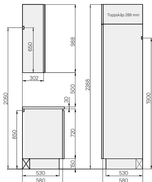
HÖJD 2388 MM
