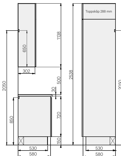
HÖJD 2538 MM
